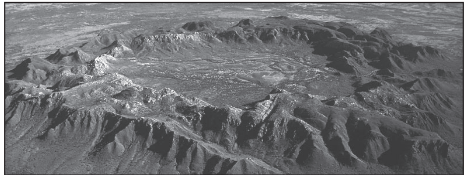
Gosses Bluff, Ausztrália, Északi Territórium. Triász időszi aszteroida-becsapódás (Dietz, 1975)
