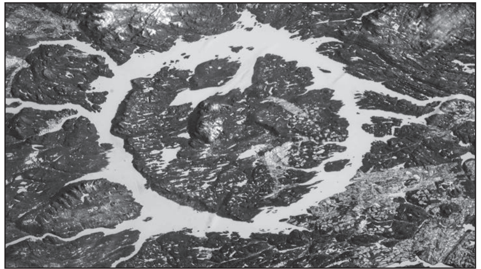
Manicouagan. Aszteroida-becsapódás a triász időszakból, a Szent-Lőrinc folyó torkolatánál, Kanadában. Téli úrfelvétel. Wikipedia
