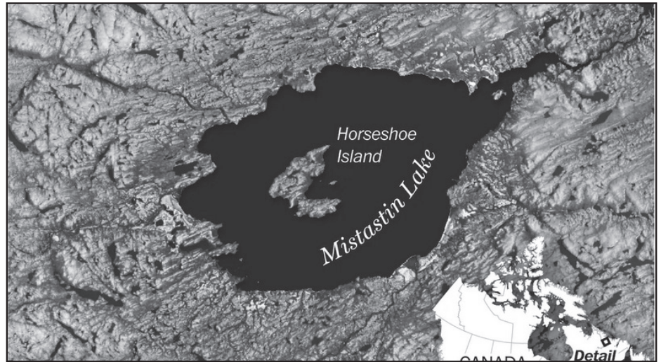
Mistastin-tó. Észak-Labrador, Új-Fundland. LANDSAT-felvétel
